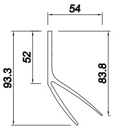
Vinastar 518 THK. 3.0mm - 1.445Kg/m
