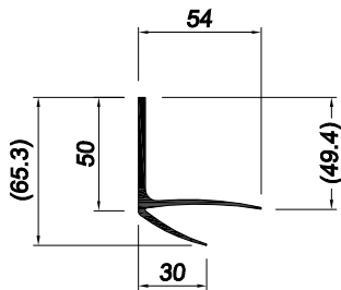
Vinastar 470 THK. 3.00 mm - 0.851 Kg/m
