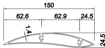
VINASTAR 060ST0105 THK. 1.40 mm - 1.375 Kg/m
